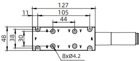
BV50 尺寸图
