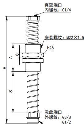
K22 吸盘连接处外螺纹
