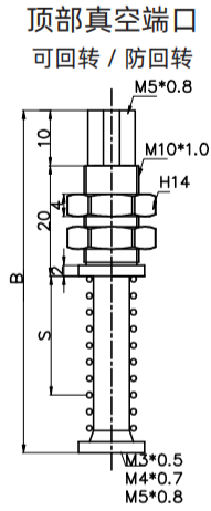
外形尺寸图 (M10)
