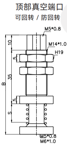
外形尺寸图 (M14)
