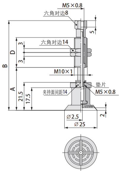
外形尺寸图 -PT 薄型缓冲式组件 (Ø25)
