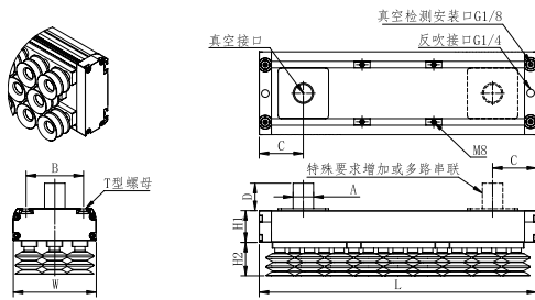
3F : 三排孔椭圆形吸附孔
