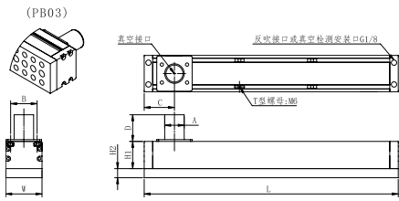
PB03：三排圆形吸附孔
