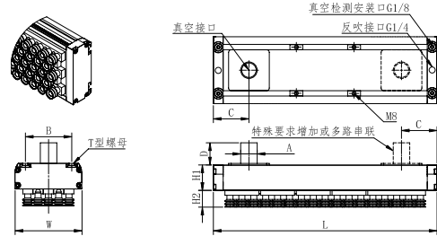
4F : 五排孔圆形吸附孔
